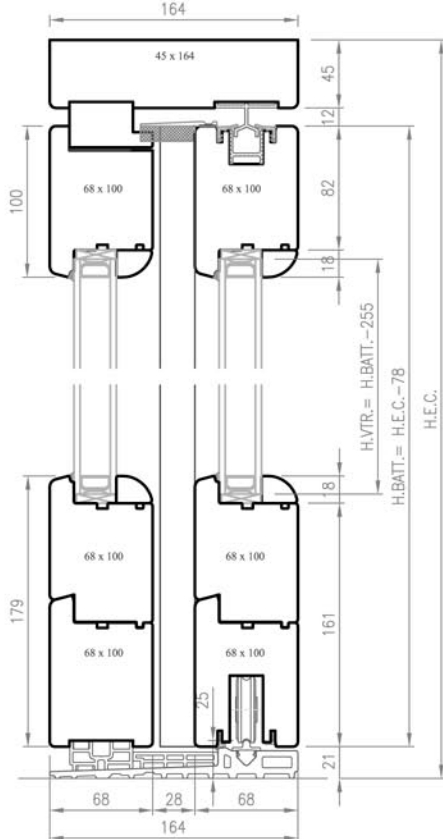
SEZ. VERTICALE
