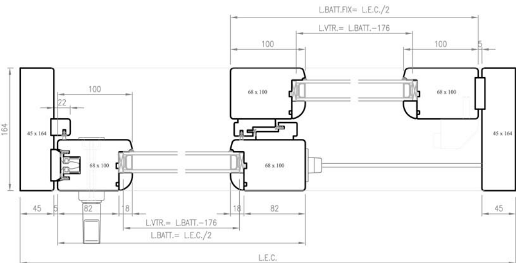
SEZ. ORIZZONTALE
